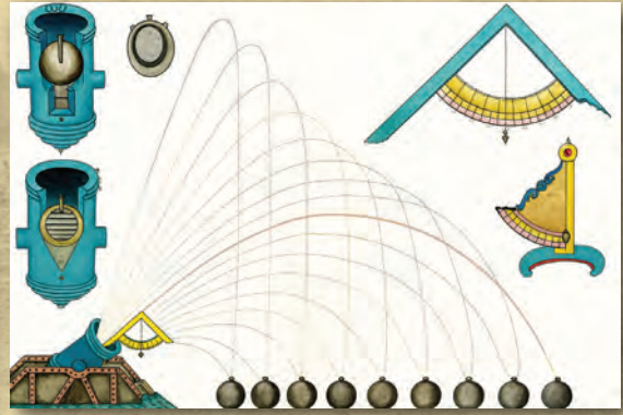
Humbaracı Ocağı'nda okutulan Fünûnî'l-Harb adlı eserdeki havan topu ve humbara çizimleri
