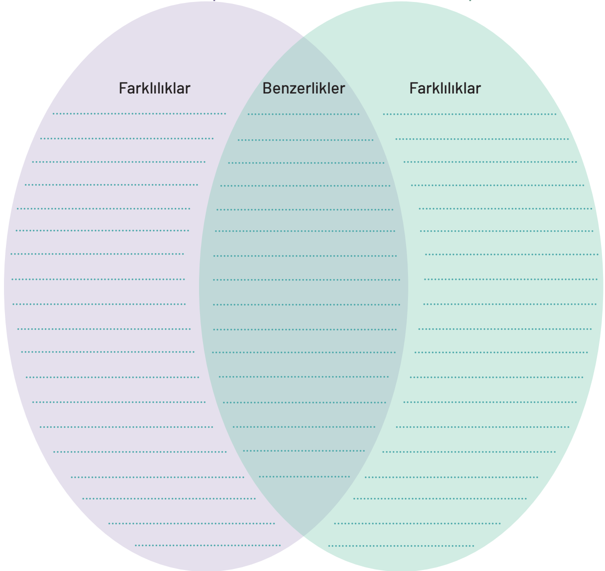
1755 Lizbon Depremi
