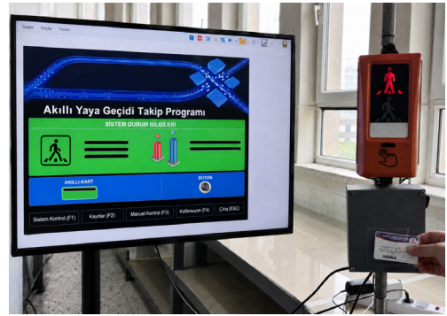
Yaya Geçitlerinde Takip Tabanlı Akıllı Yaya Geçidi Sinyal Sistemi Ekranı
