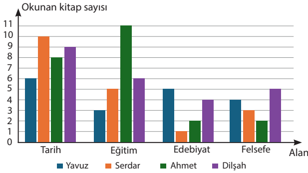
Grafik 1: Öğrencilerin türlere göre okudukları kitap sayılarını gösteren sütun grafiği
