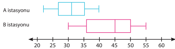
Grafik 3: A ve B istasyonlarından yaktı alan araba sayılarına ait kutu grafikleri
