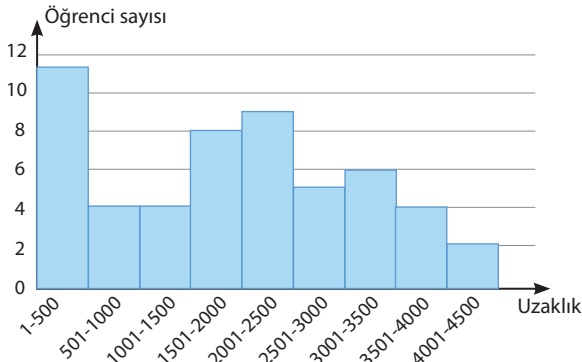
Grafik 5: Bir sınıftaki öğrencilerin evlerinin okula uzaklıklarını gösteren histogram
