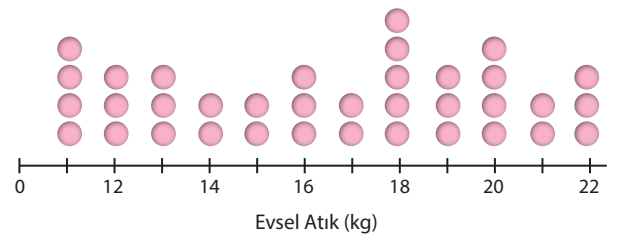
Grafik 6: Bir sitede yaşayan ailelerin haftalık evsel atık miktarlarını gösteren nokta grafiği
