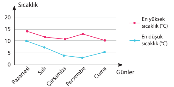
Grafik 4: Bir ildeki 5 günlük tahmini hava sıcaklığını gösteren çizgi grafiği
