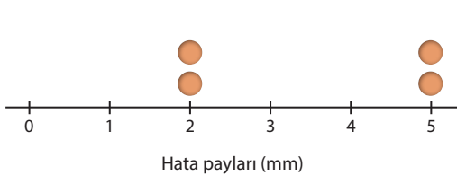
Grafik 1: A makinesinin hata payları
