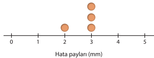
Grafik 2: B makinesinin hata payları
