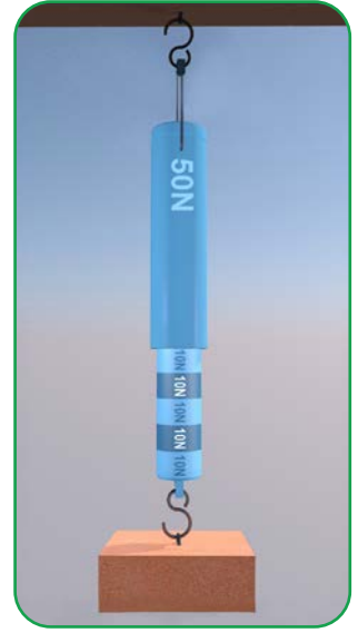
Görsel 2.1.8: Ölçebileceği kuvvet değeri ve bölme sayısı verilen dinamometre
