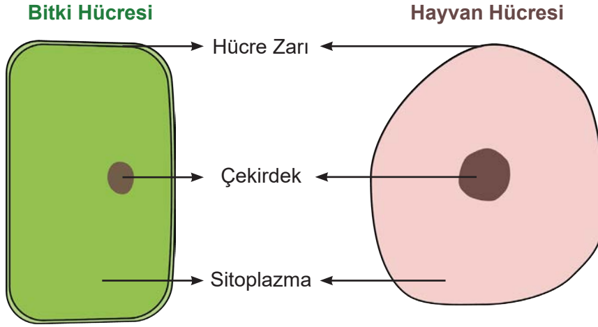
Görsel 3.1.15: Hücrenin temel kısımları
