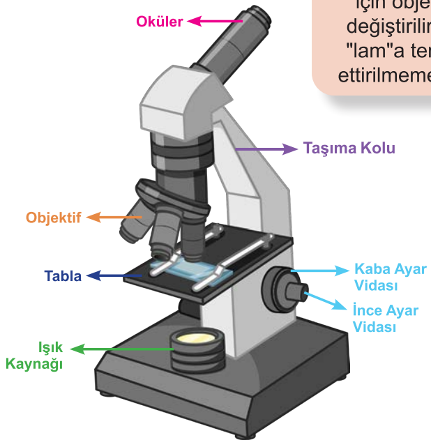
Görsel 3.1.2: Mikroskopun bölümleri
