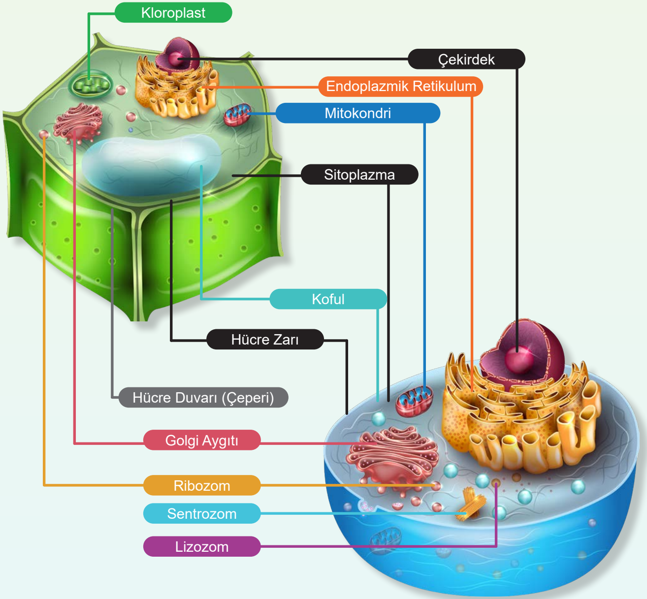
Görsel 3.1.13: Bitki ve hayvan hücresi
