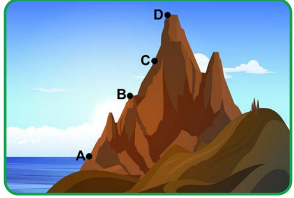
Görsel 2.2.8: Yeryüzündeki farklı konumlar
