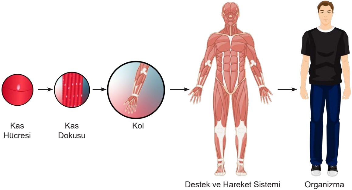
Görsel 3.1.17: Hücreden organizma oluşumu
