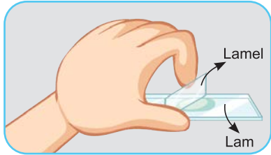
Görsel 3.1.1: Örnek hazırlanışı
