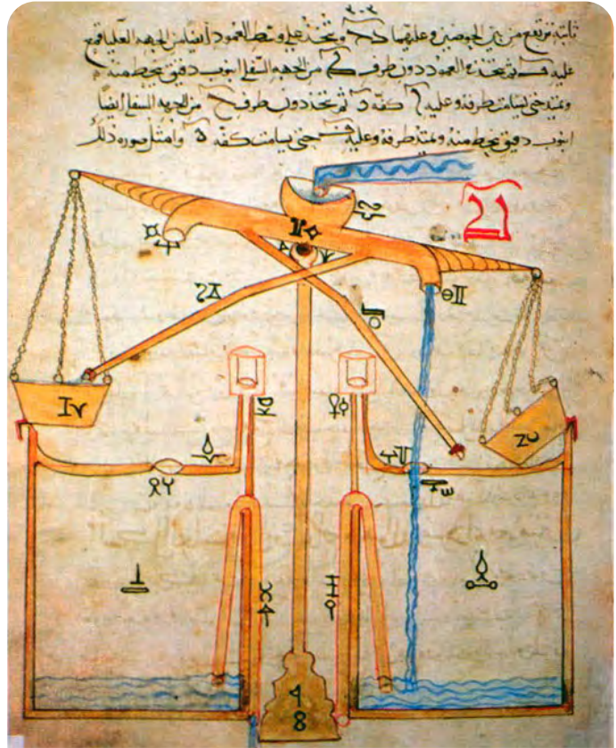
Görsel 1.5: Cezeri'nin icat ettiği iki şamandıralı fiskeye
